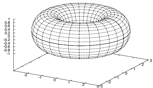
Figura 8.6 Toro
