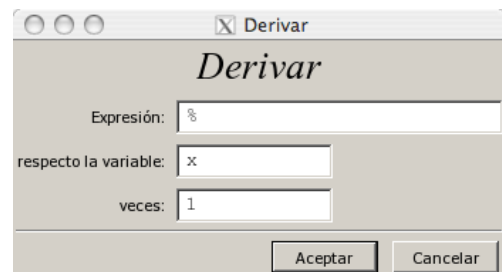
Figura 6.1 Introducir derivada
