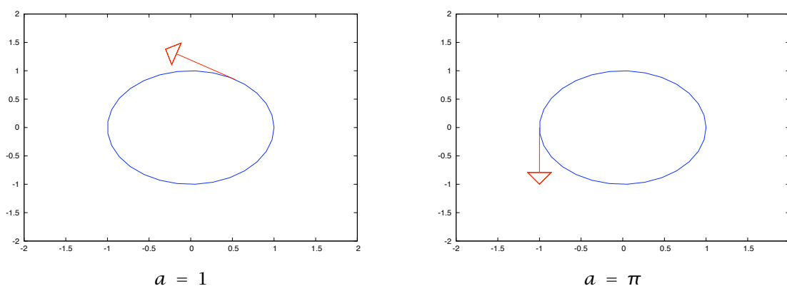
Figura 10.1 Curva y vectores tangentes
