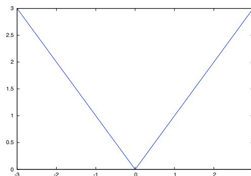
Figura 10.2 ¿Es diferenciable?
