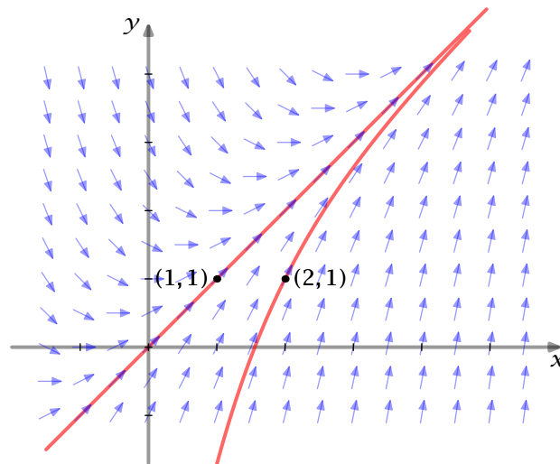
Figura 9.1 Campo de pendientes y curvas integrales
