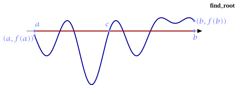
Figura 4.1 Teorema de los ceros de Bolzano
