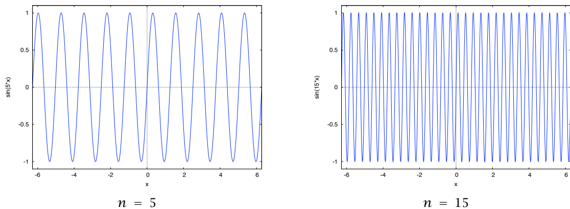
Figura 2.6 \sin(nx)
