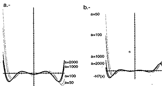
Figura 3: Límite (29) para diferentes a y n = 10 .
