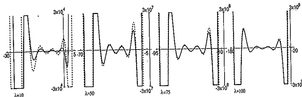
Figura 16: Aproximación (102) para n = 10 . La línea discontinua representa P_{10}^{(\lambda)}(x, \phi) , la línea continua z^{10}C_{10}(\xi, C)/10!
