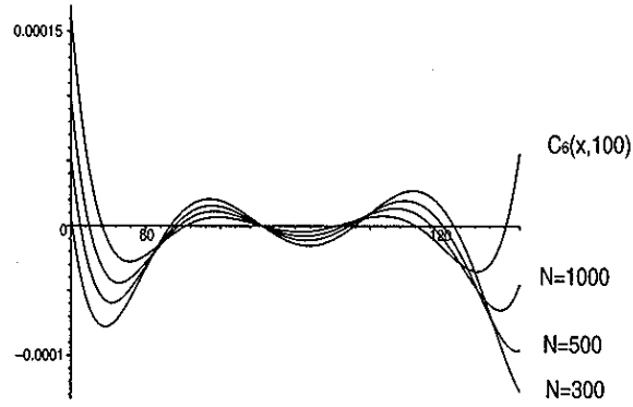
Figura 14: Límite (87) para n = 5 .
