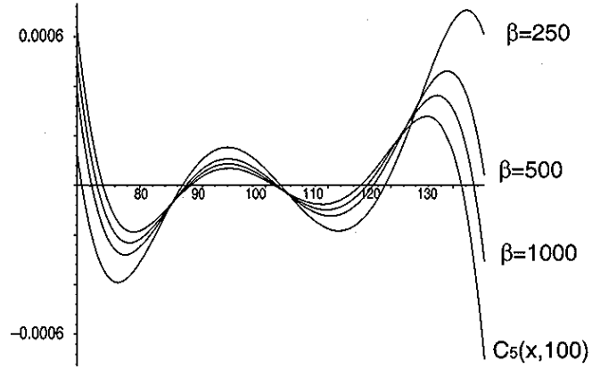
Figura 12: Límite (72) para n = 5 .
