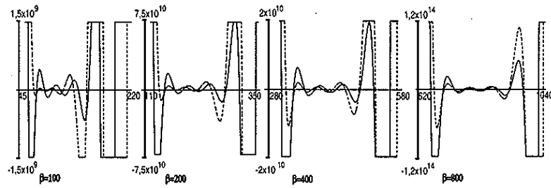
Figura 6: Aproximación obtenida con el primer término de (38) para n = 10 y c = 1/2 . Las líneas continuas representan M_{10}(x; \beta, c) . Las líneas discontinuas representan la aproximación z^{10}H_{10}(\xi)/10! .
