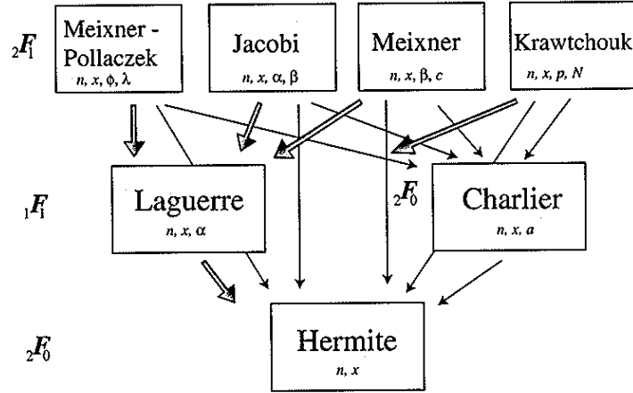
Figura 1: Tres últimos niveles de la tabla de Askey de los polinomios hipergeométricos ortogonales. Las flechas gruesas indican relaciones asintóticas conocidas entre los polinomios que conectan, mientras que las flechas finas indican nuevos desarrollos asintóticos obtenidos en este trabajo.
