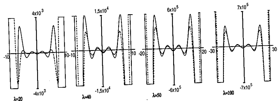
Figura 8: Aproximación obtenida con el primer término de (44) para n = 10 y \phi = \pi/2 . Las líneas continuas representan P_{10}^{(\lambda)}(x; \phi) . Las líneas discontinuas representan la aproximación z^{10} H_{10}(\xi)/10! .
